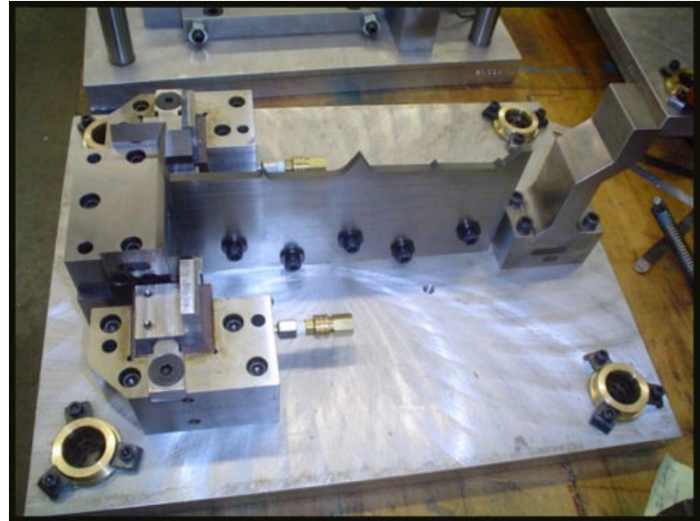
Notch & Shear Die
